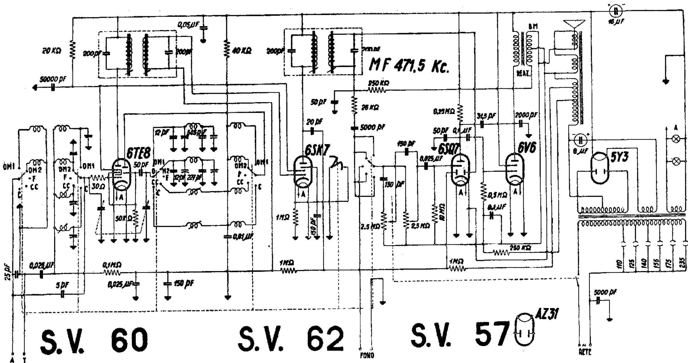
MAGNADYNE RADIO - Modd. SV 57, SV 60, SV 62 - Gamma onde medie divisa e due gamme onde corte. Media frequenza 471,5 kc/s. Il mod. SV 57 differisce per avere la raddrizzatrice AZ31 al posto della 5Y3. Potenza d'uscita 4 W. Consumo 60 W circa.
